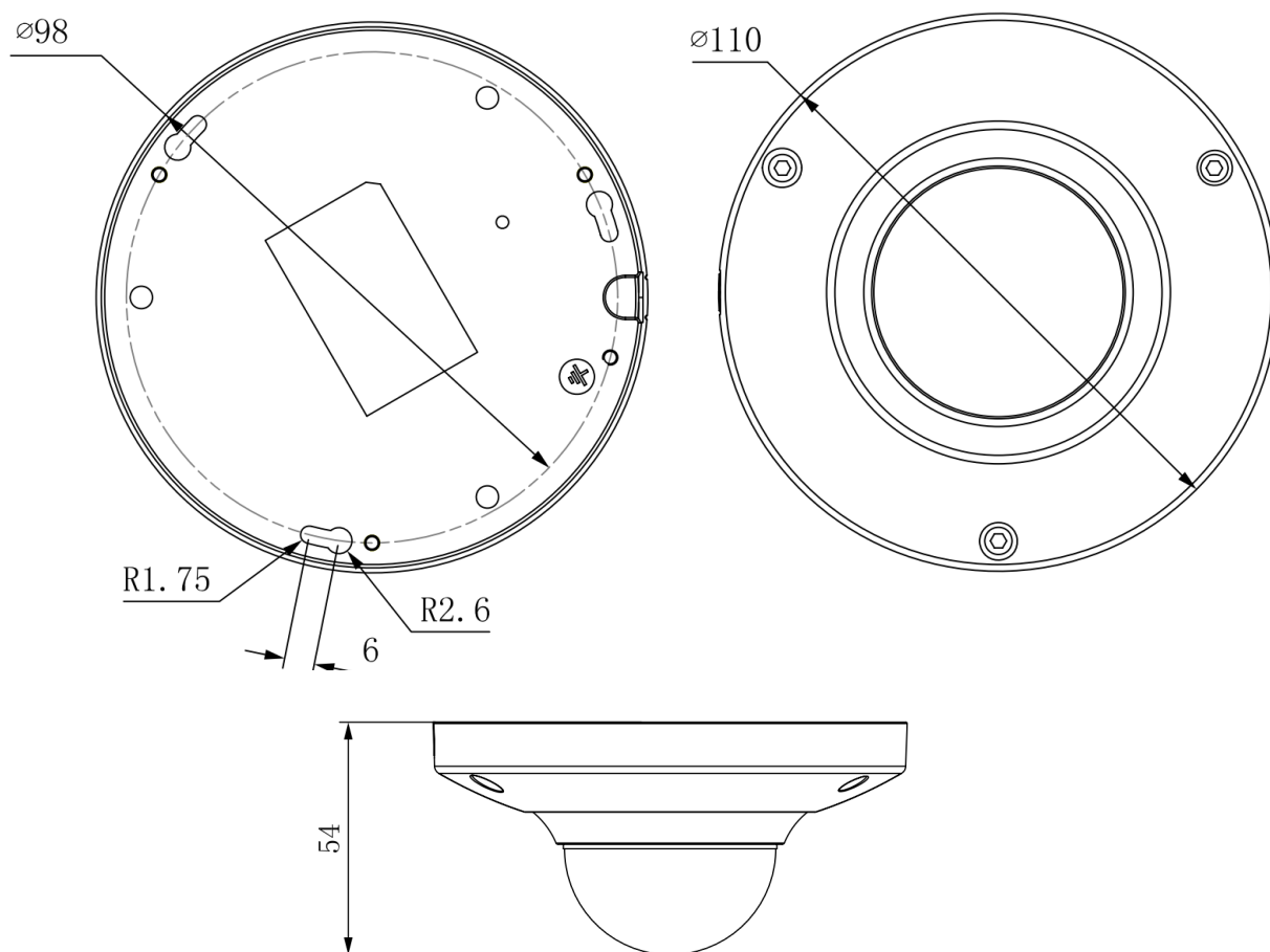
Рис. 1.1. Внешний вид и размеры
